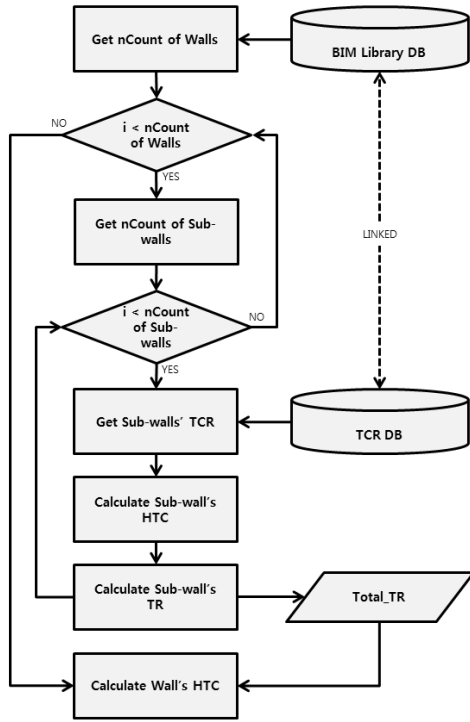
그림7. 열관류율 추출 알고리즘의 순서도(TCR: 열전도율, TR: 열저항, HTC: 열관류율)
